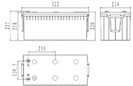
外形尺寸
